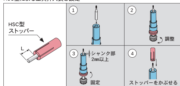
HSC型による工具挿入長さ設定
