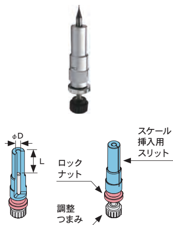
HSC型による工具挿入長さ設定
