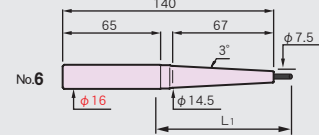
ST16-SLRA3-140-M67
