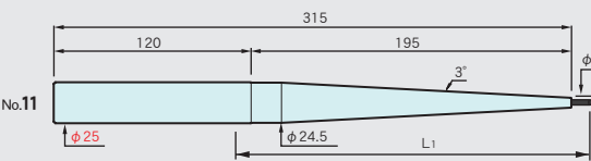
ST25-SLSA3-315-M195
