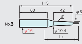
ST16-SLSA3-115-M42
