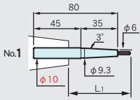
ST10-SLSA3-80-M35
