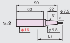
ST16-SLRA3-90-M22
