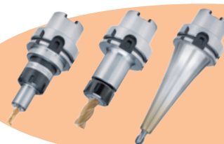
ミーリングツール Milling tool ●HSK-A63
