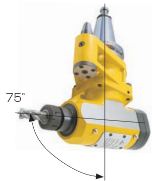
75度 角度头 75 degree angle
